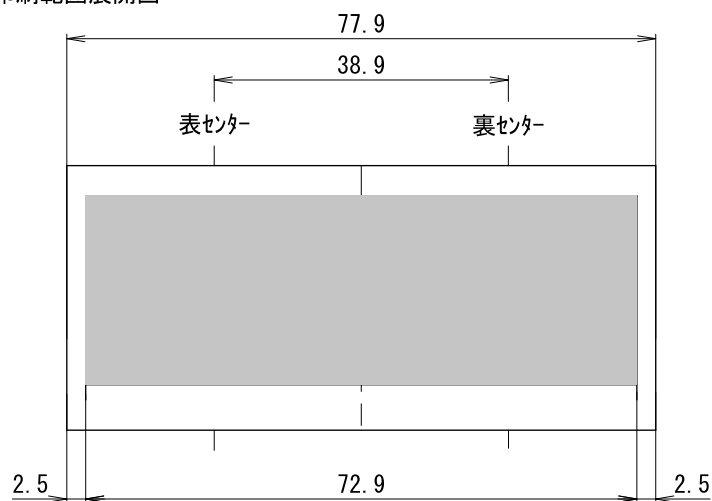
印刷範囲展開図
