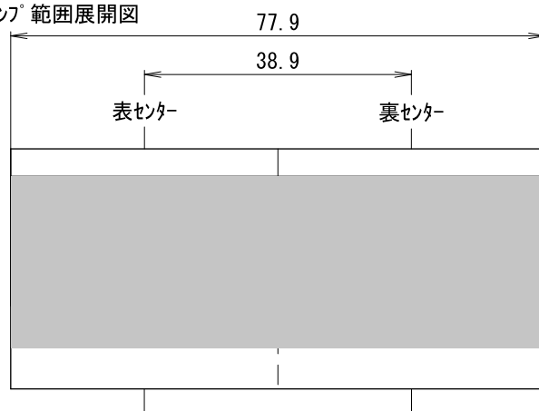
ホットスタンプ 範囲展開図
