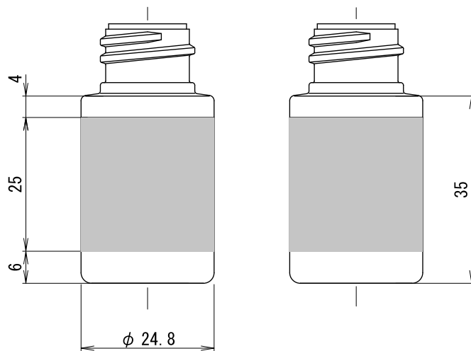
印刷範囲展開図
